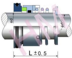
HMFR-02-A+D(Vulcan W-XX08/12)
